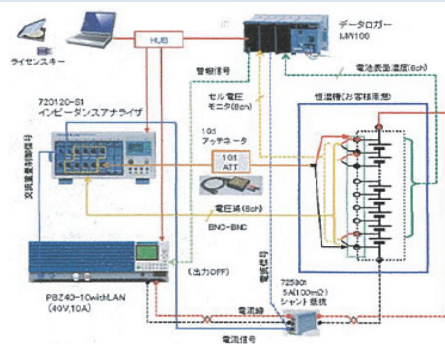
図 モジュール電池用診断器プロトタイプの計測システム
